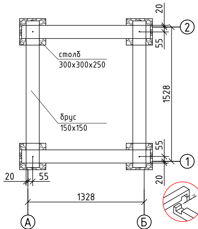
Пример схемы фундамента на столбах
